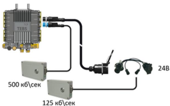
Варианты подключения для блоков с модулем CAN 24
