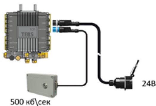
Вариант подключения для блоков без модуля CAN 24
