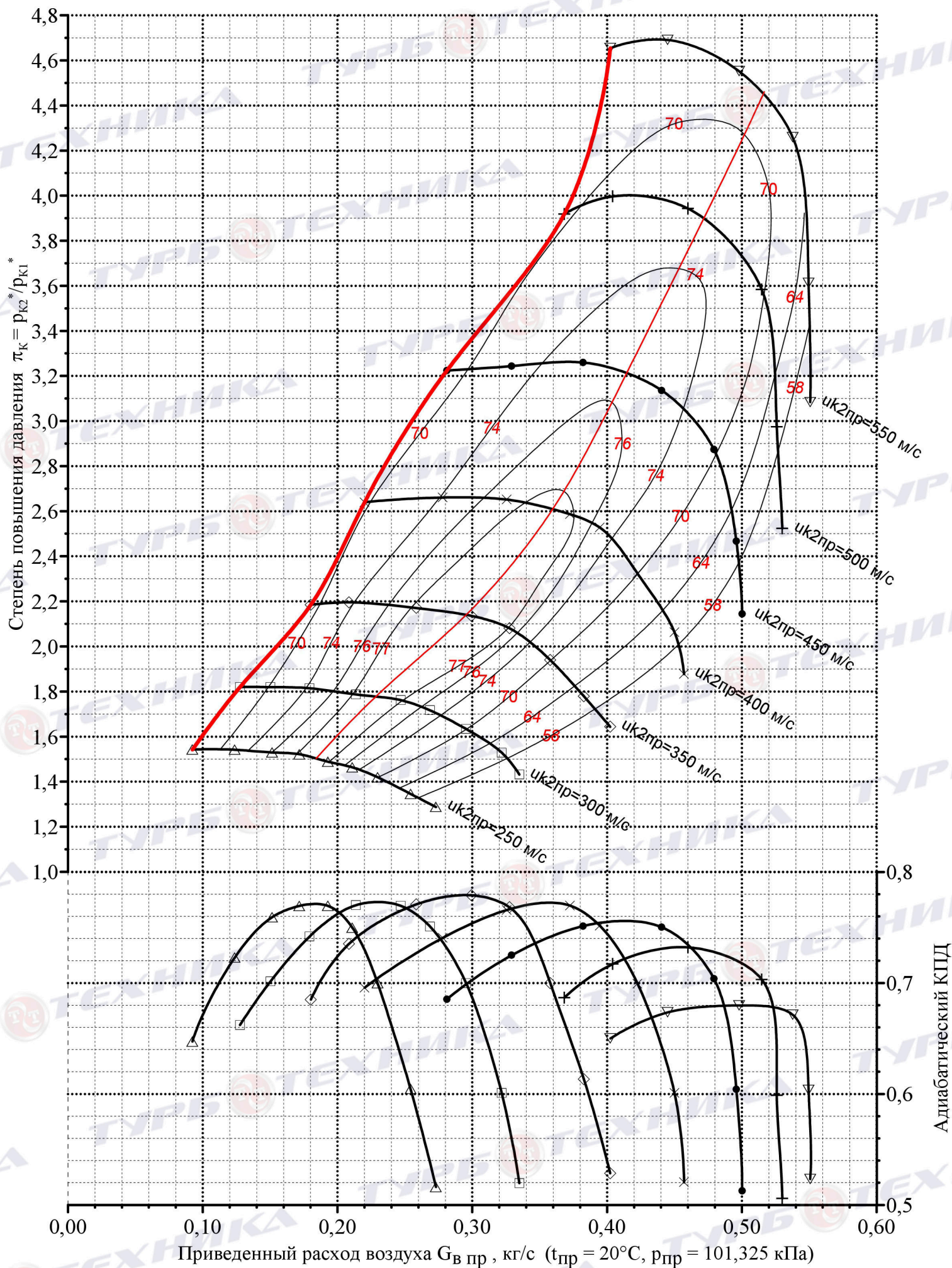
ХАРАКТЕРИСТИКИ КОМПРЕССОРА ТКР 90.06.15
